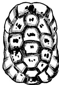
Kappa Shell
