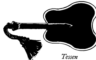
Tessen
